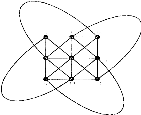
AG(2,3) .
