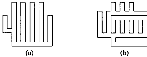
Figure 4: A Hamilton cycle for : (a) R(11, 12)^{-3(3,2)} (b) R(11, 12)^{-3(2,3)}
